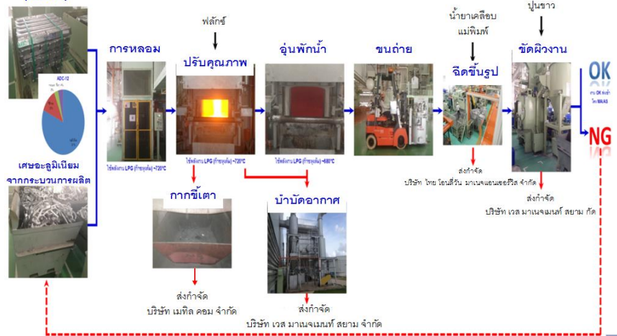
ภาพที่ 6 ภาพแสดงกระบวนการผลิตอาคารอัดกึ่ง/ประกอบและฉีดขึ้นรูปพลาสติก
